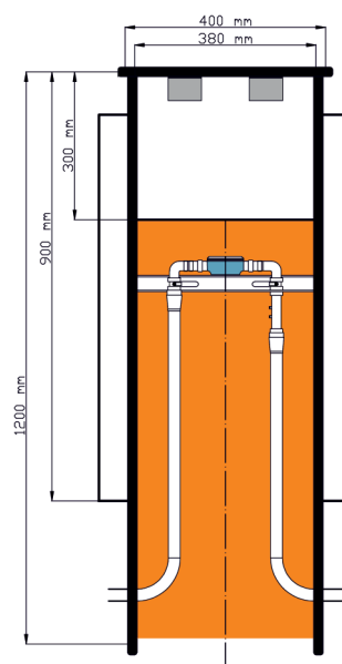
STUDNIA AS1 Z PRZYŁĄCZEM KOLANKOWYM W ŚCIANCIE
